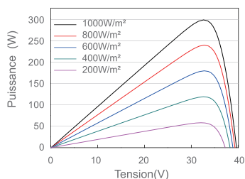
Courbe puissance-tension JAM60S02-300/PR
